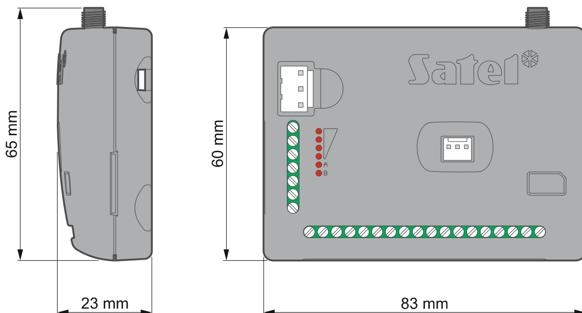
Obr. 5. Rozměry krytu modulu GPRS-A LTE.
