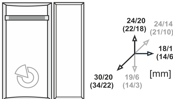
Obrázek 2: vzdálenosti pro aktivaci /deaktivaci detektoru montovaném na nemagnetickém (magnetickém) podkladu
